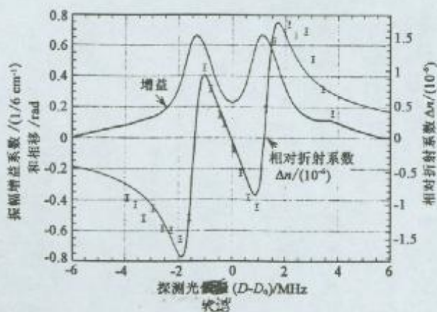
图 1 使用一束可调频的连续激光测得的铯原子气体中,光波振幅的增益系数以及折射指数随光波频率的变化曲线
